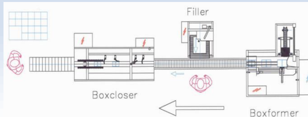
Aufstellungsvorschlag mit Handfüller A1001
