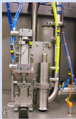
Chambre de remplissage
